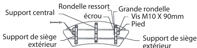
Vue de dessous du siège
