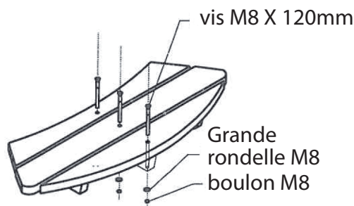
Vue du dessus du siège
